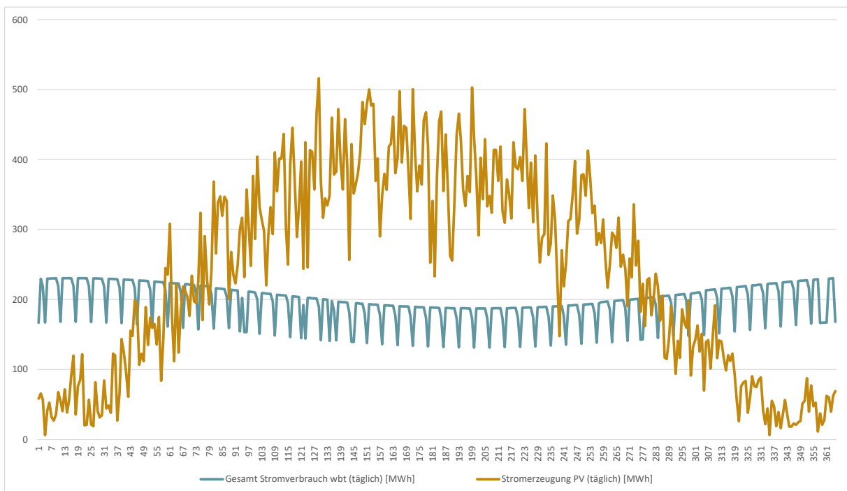
Abbildung 26 Vergleich zwischen Stromerzeugung und -verbrauch (täglich) für das Klimaschutzszenario in 2040
