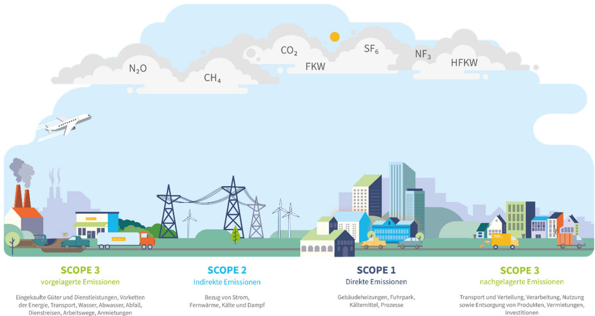
Abbildung 46 Wirkungsbereiche (Scopes)
